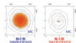
宇宙線で捉えた太陽の影。磁場の影響により、極小期はくっきり映り、極大期には見えなくなる。
